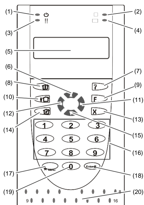
Figuur 1: ATS111xA-gebruikersinterface
