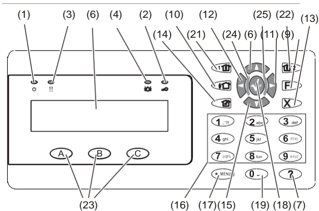
Figuur 2: ATS1135-gebruikersinterface
