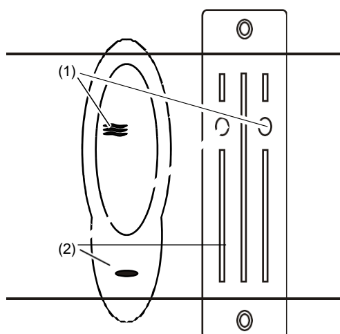
Figuur 3: ATS1190/ATS1192-lezers
